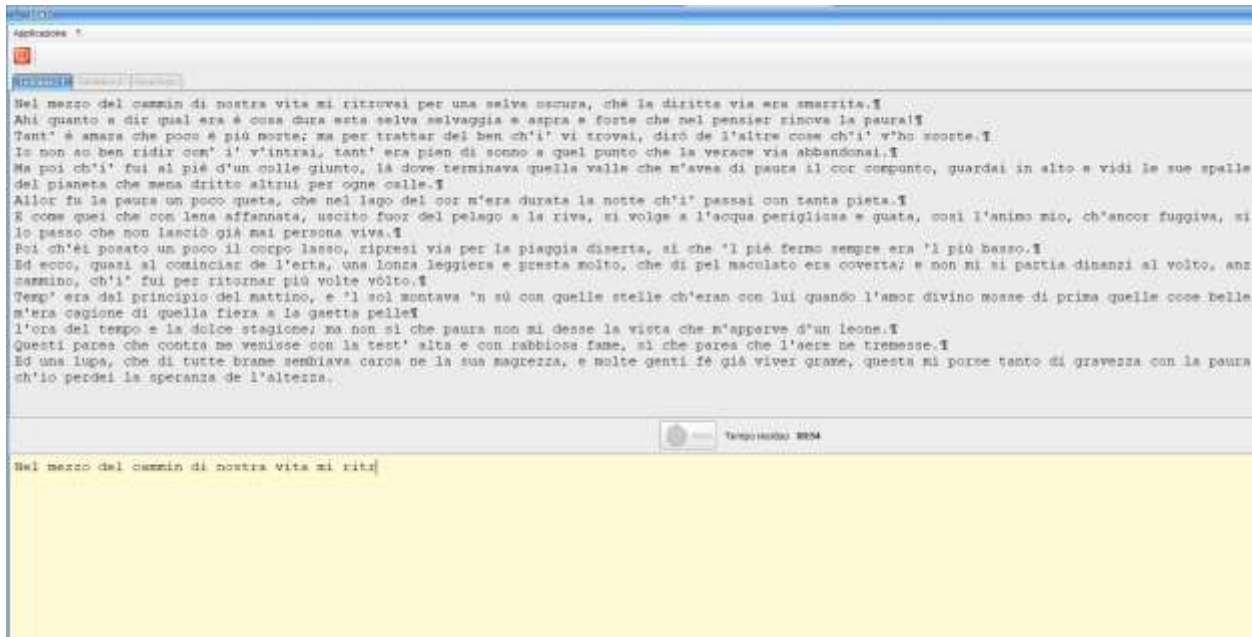
Figura 6 - Tentativo 1 avviato
