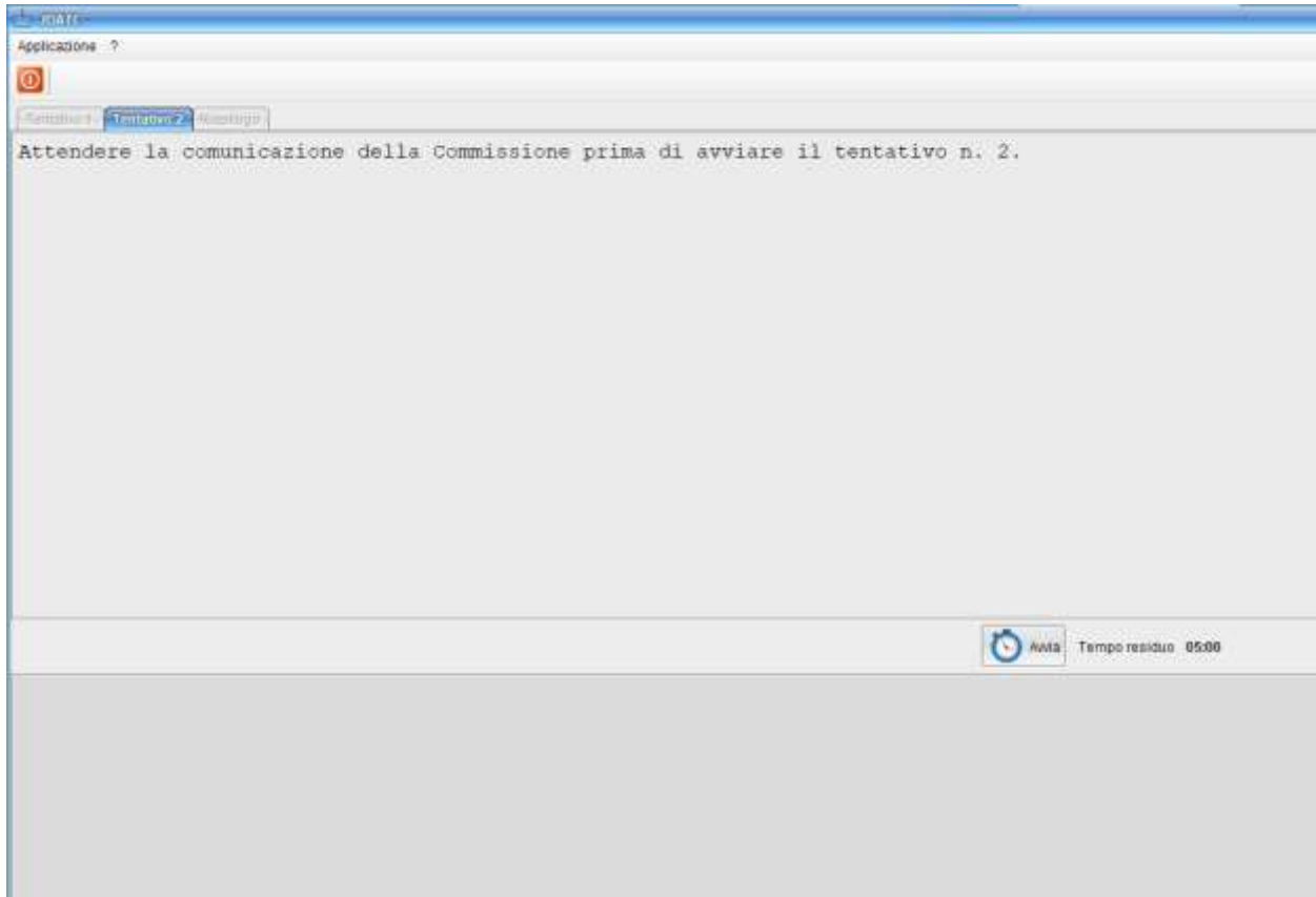
Figura 9 - Schermata Tentativo 2
